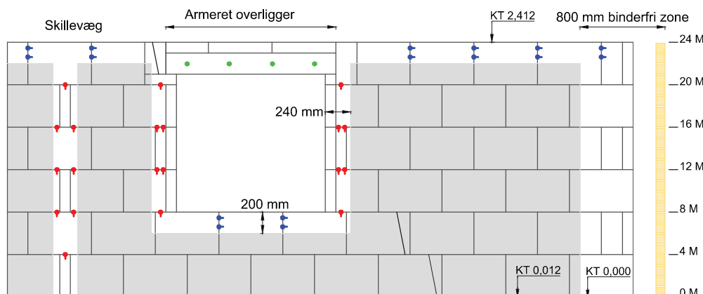
Fig. 1. Murbindere placeres jf. EC 6. I overligger og omkring muråbninger anvendes bindere til indskruning. I de grå områder fordeles bindere jf. projektmaterialet.
